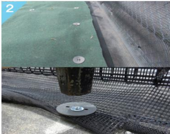
フェンス足元の処理
